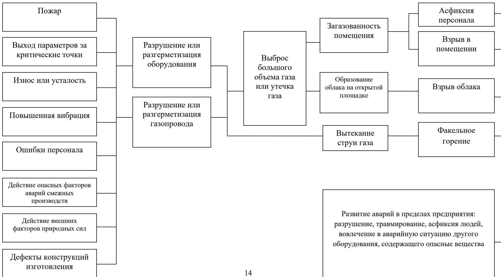
Рисунок 1. Блок-схема сценариев возникновения аварийных ситуаций на котельной пос. Лесосплава, д. 28, г. Кольчугино
